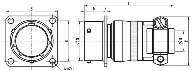
Square flange receptacle with cable clamp backshell. Embase à collerette carrée avec raccord serre-câble.
